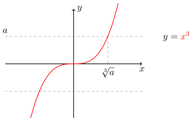
Obrázek 4.8: Konstrukce liché odmocniny čísla a .
