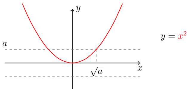
Obrázek 4.6: Ke konstrukci sudé odmocniny čísla a .
