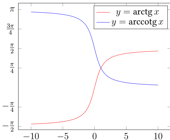
Obrázek 4.14: Grafy funkcí \arctg x a \operatorname{arccotg} x .
