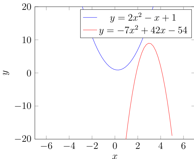
Obrázek 4.5: Ukázka grafů dvou kvadratických funkcí.
