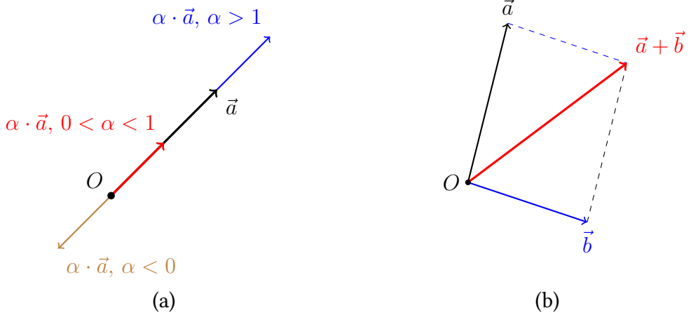
Obrázek 5.2: Geometrický význam násobení vektoru číslem (a) a sčítání vektorů (b).
