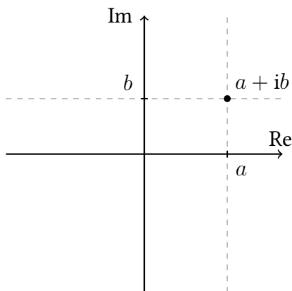
Obrázek 3.5: Komplexní rovina.
