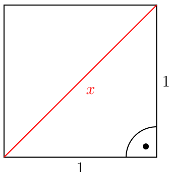
Obrázek 3.3: Čtverec o straně délky 1 a jeho úhlopříčka o straně délky x .
