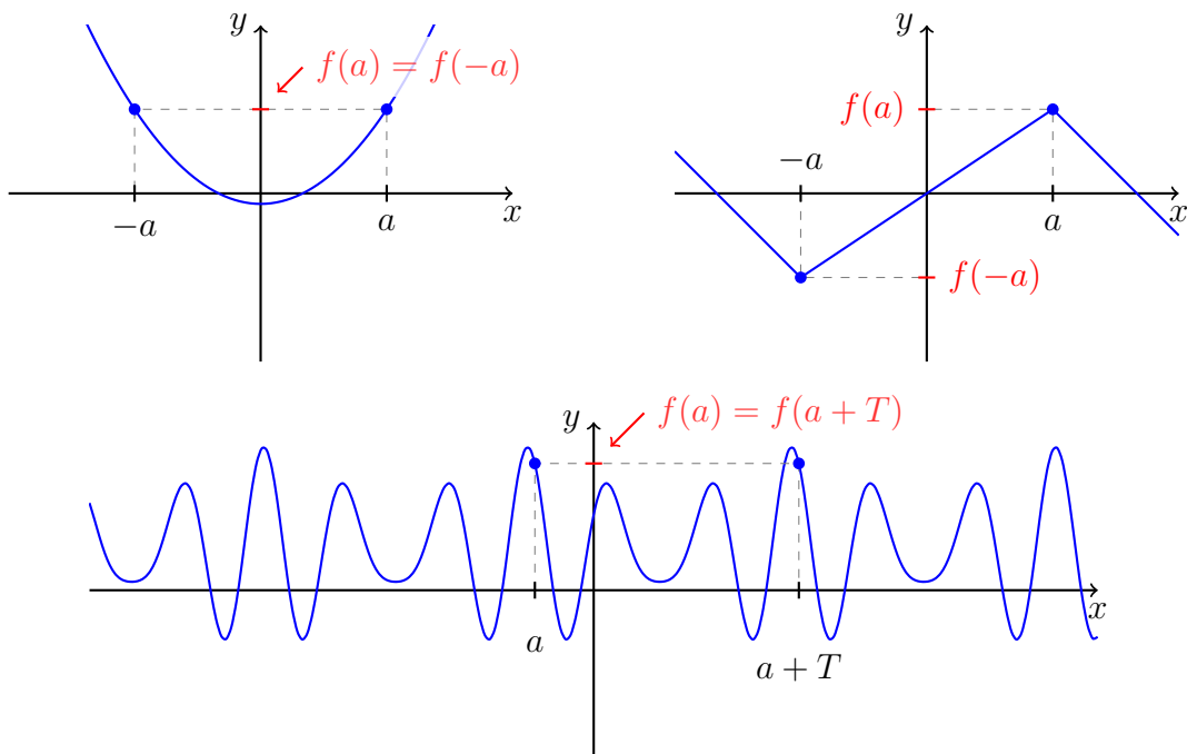
Obrázek 4.1: Grafické znázornění sudosti, lichosti a periodicity v definici č. 4.4 (popořadě).
