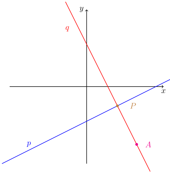
Obrázek 5.3: K odvození vzorce pro vzdálenost bodu A od od přímky p .
