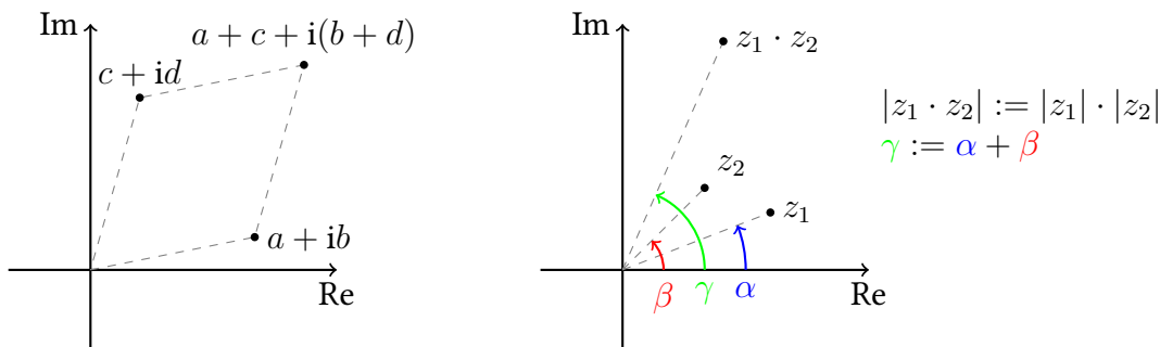
Obrázek 3.6: Geometrická interpretace operace sčítání a násobení komplexních čísel.
