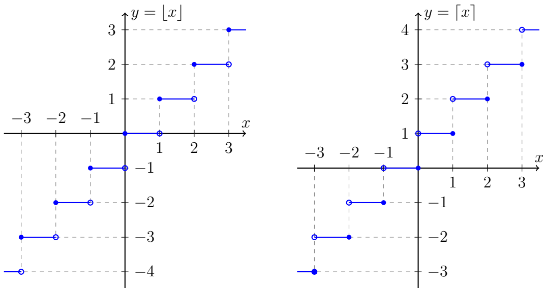
Obrázek 4.3: Grafy dolní (vlevo) a horní (vpravo) celé části.
